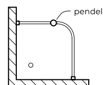
L-vormig (douche)
