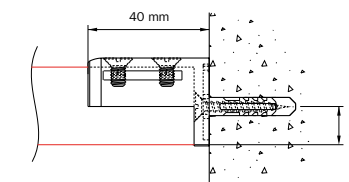
Wandmontage 5100 met dagsteun 5149
