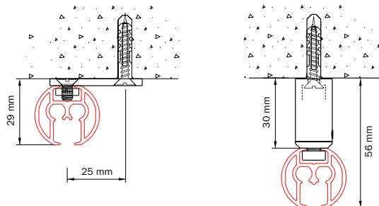
Plafondmontage 5100 met plafondsteun 5135
